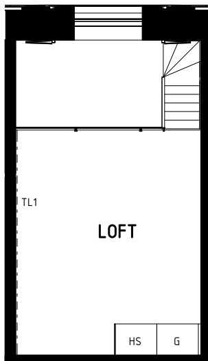
ÖVRE PLAN
